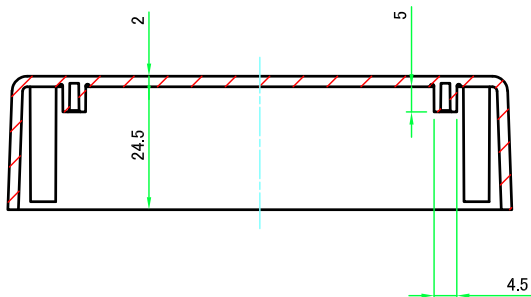
E-E ( 1 : 1.5 )
